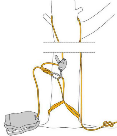
Fig. 5 - Ancoraggio della fune con dispositivo passante
