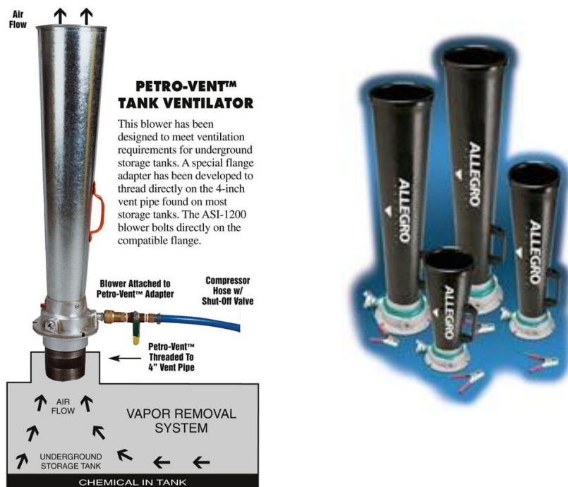
Fig. 26. Eiettori ad aria compressa, pensati per ambienti particolari. Si notino nell'immagine di destra le pinze per il collegamento equipotenziale ,contro i fenomeni elettrostatici. PRODUTTORE Allegro http://www.allegrosafety.com/
